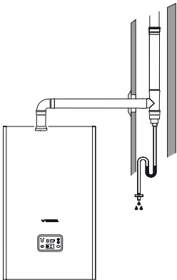
Dimensioni interne minime del cavedio per il passaggio di n° 1 tubo fumi da 50 mm di diametro
