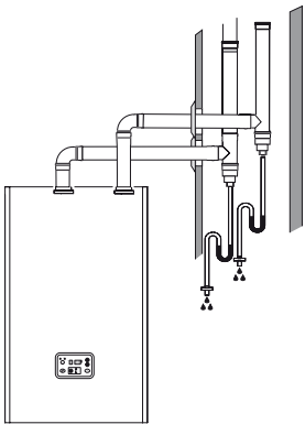
Dimensioni interne minime del cavedio per il passaggio di n° 2 tubi fumo da 50 mm di diametro
