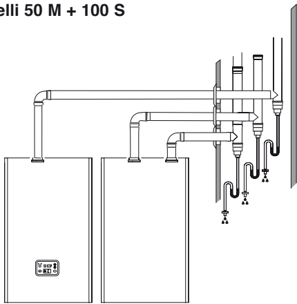
Dimensioni minime del cavedio per il passaggio di tre tubi fumo da 50 mm di diametro
