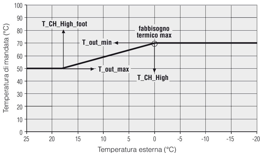
CURVA CLIMATICA Circuito ALTA TEMPERATURA
